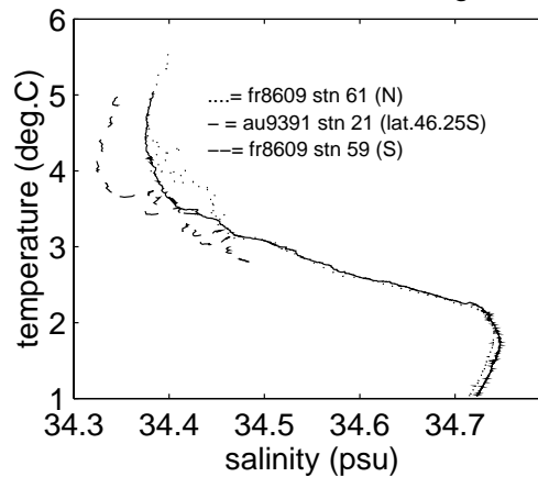
(d) 1000 to 2000 dbar TS diagram
