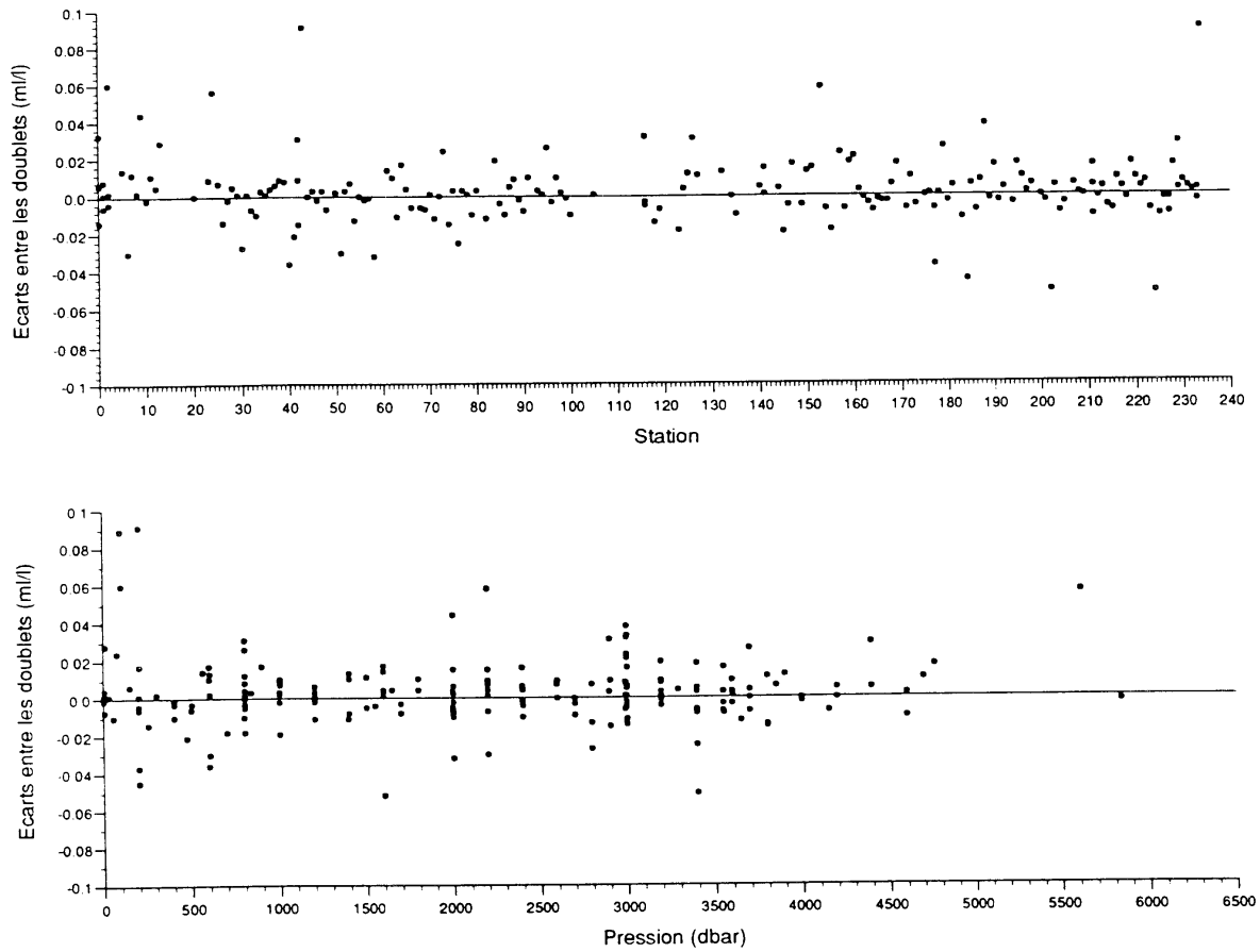
Figure III-5: Écarts en oxygène entre deux bouteilles fermées au même niveau: Σ en fonction du numéro de station à laquelle est réalisé le doublet, Σ en fonction de la pression à laquelle est réalisé le doublet.
