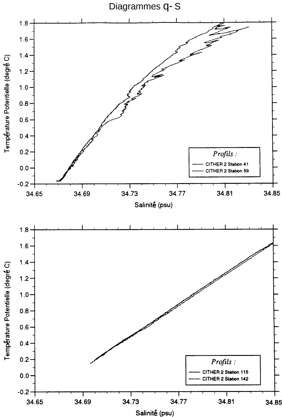
Figure 17: Comparaison de diagrammes q- S tracés d'après les données de la campagne CITHER 2.
