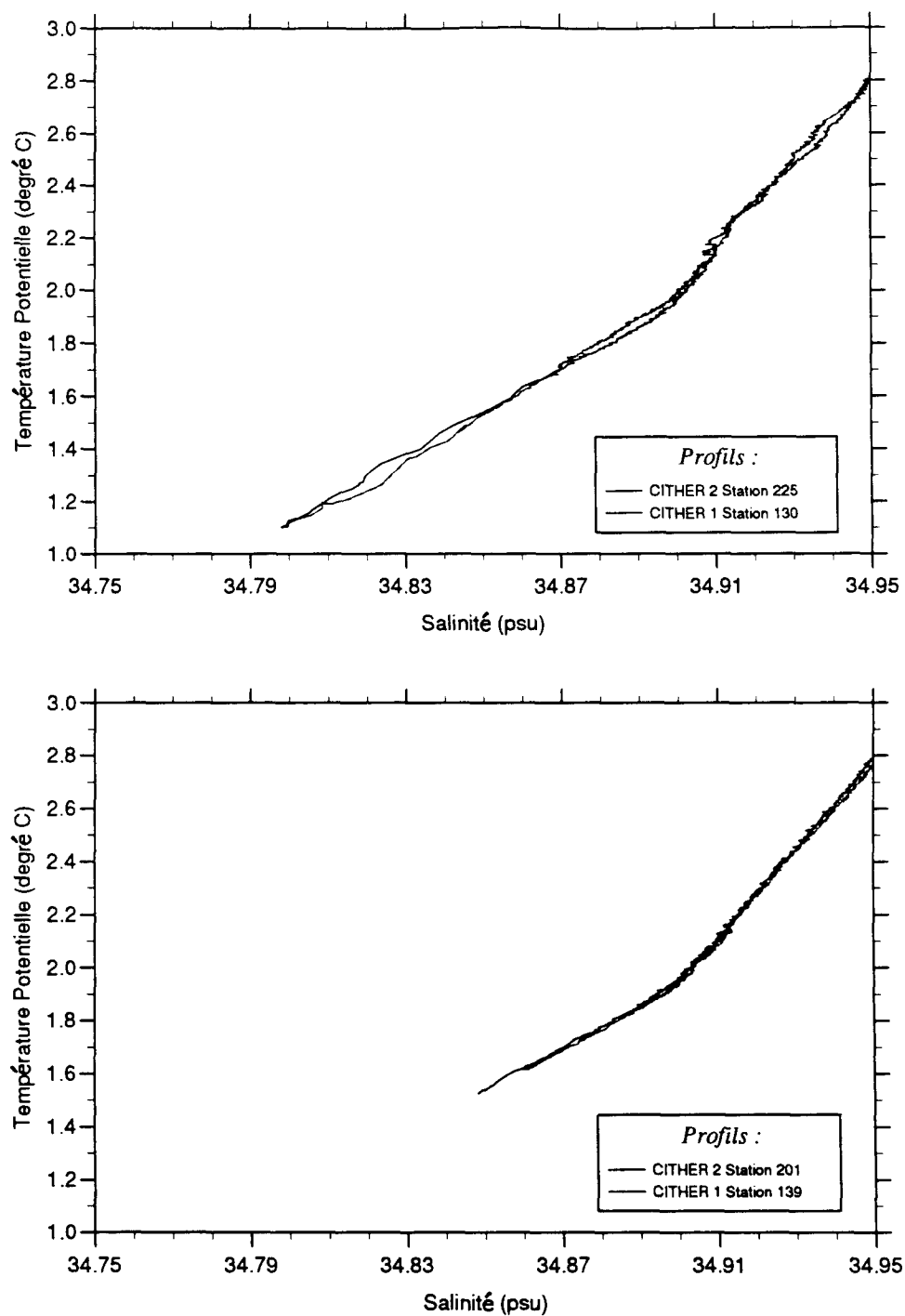
Figure 18: Comparaison de diagrammes Q- S de la campagne CITHER 2 avec les données d'autres campagnes obtenues à une position géographique proche: a) station 225 de CITHER 2 et station 130 de CITHER 1 (profil CID), b) station 201 de CITHER 2 et station 139 de CITHER 1 (profil CM).
