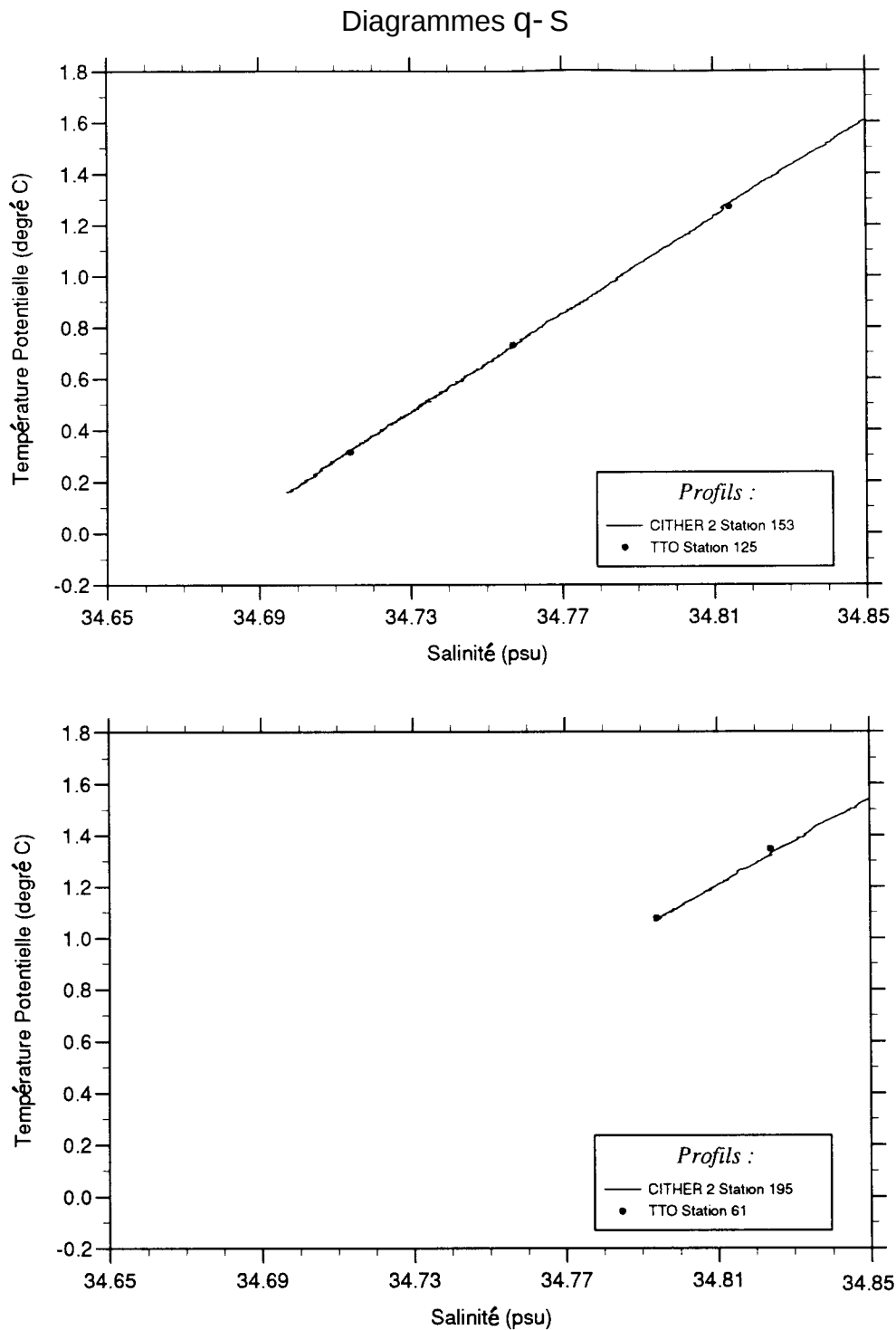
Figure 20: Comparaison de diagrammes Q- S de la campagne CITHER 2 avec les données d'autres campagnes obtenues à une position géographique proche: a) station 153 de CITHER 2 et station 125 de TTO (données "rosette"), b) station 195 de CITHER 2 et station 61 de TTO (données "rosette").
