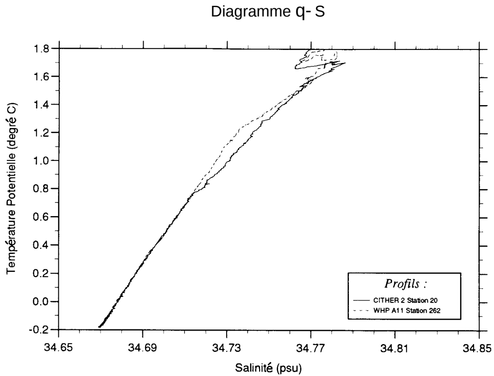
Figure 21: Comparaison de diagrammes q- S de la campagne CITHER 2 avec les données & autres campagnes obtenues à une position géographique proche:
