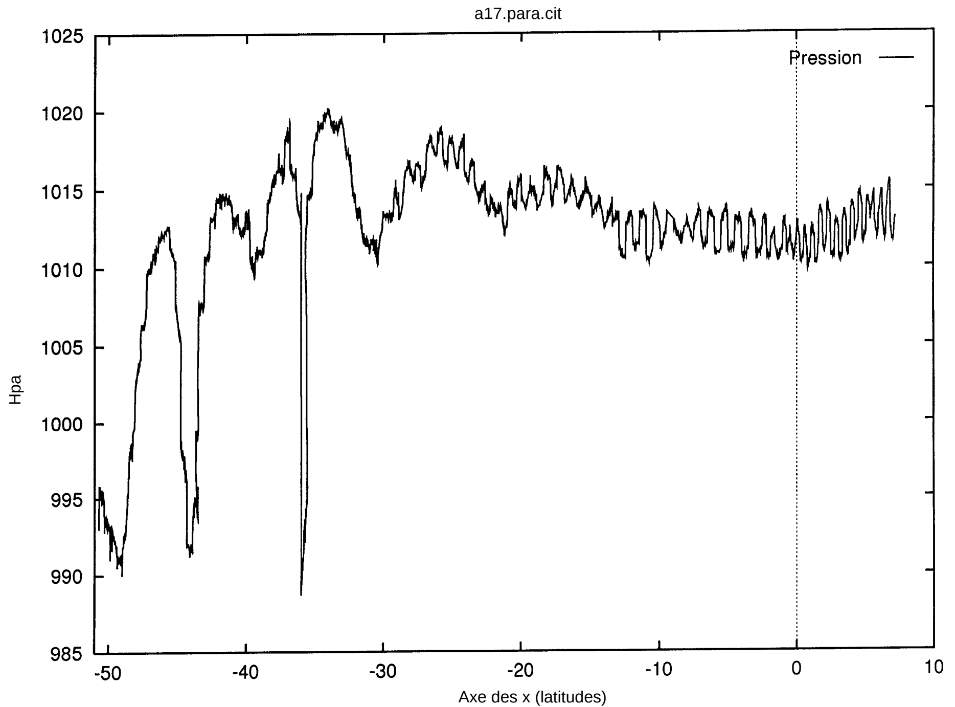
Figure V-7a: Pression atmospherique le long de la grande section A17
