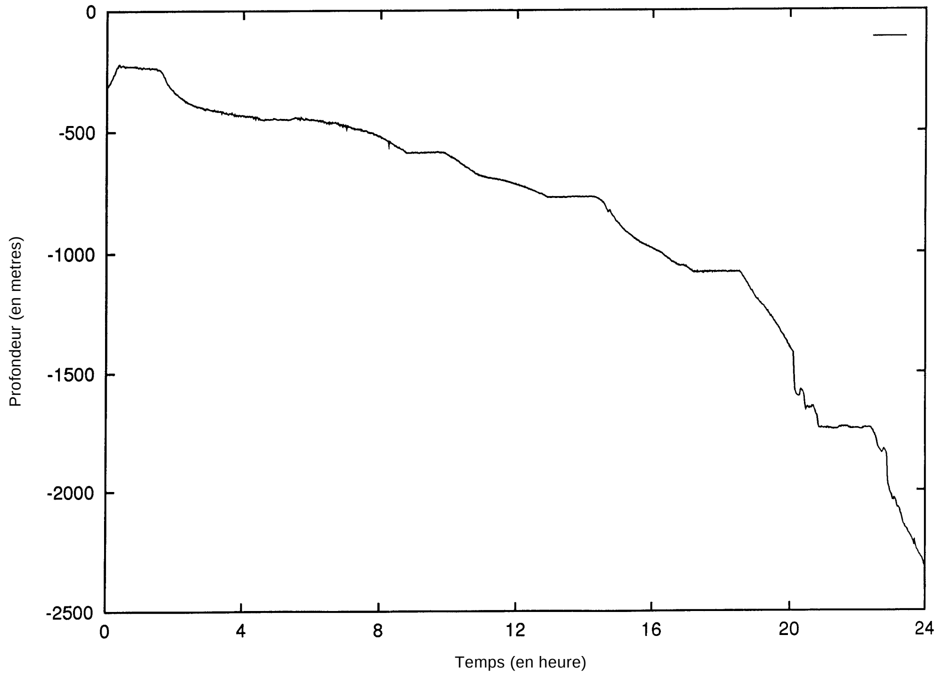
Figure V-4: Zoom sur la bathymetrie mesuree le 10/01/94
