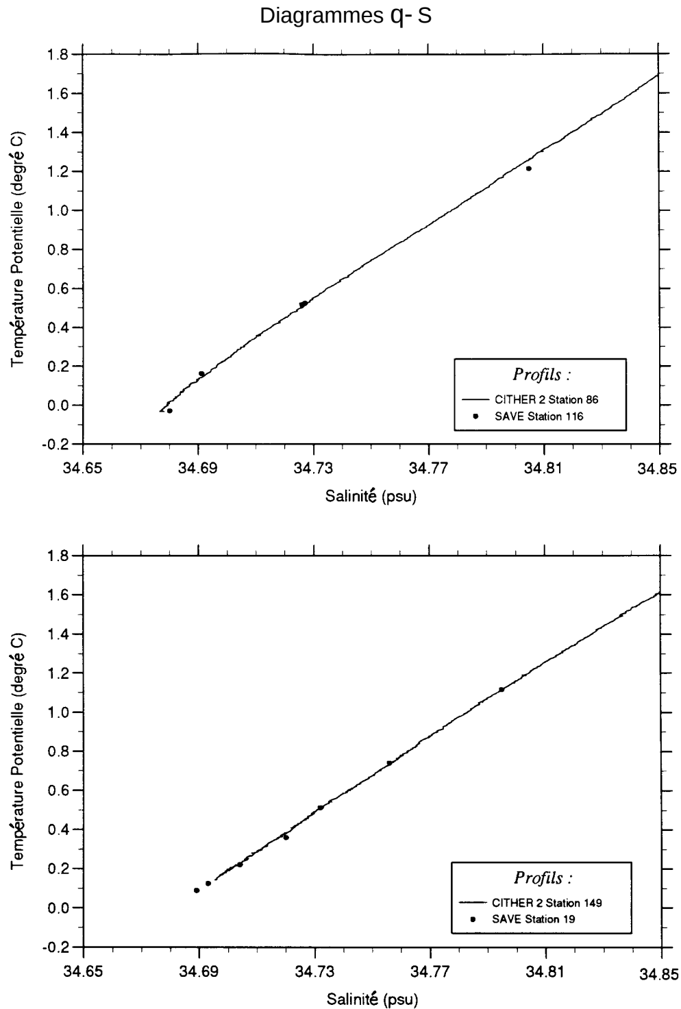
Figure 19: Comparaison de diagrammes q- S de la campagne CITHER 2 avec les données d'autres campagnes obtenues à une position géographique proche: a) station 86 de CITHER 2 et station 116 de SAVE (données "rosette"), b) station 149 de CITHER 2 et station 19 de SAVE (données "rosette").
