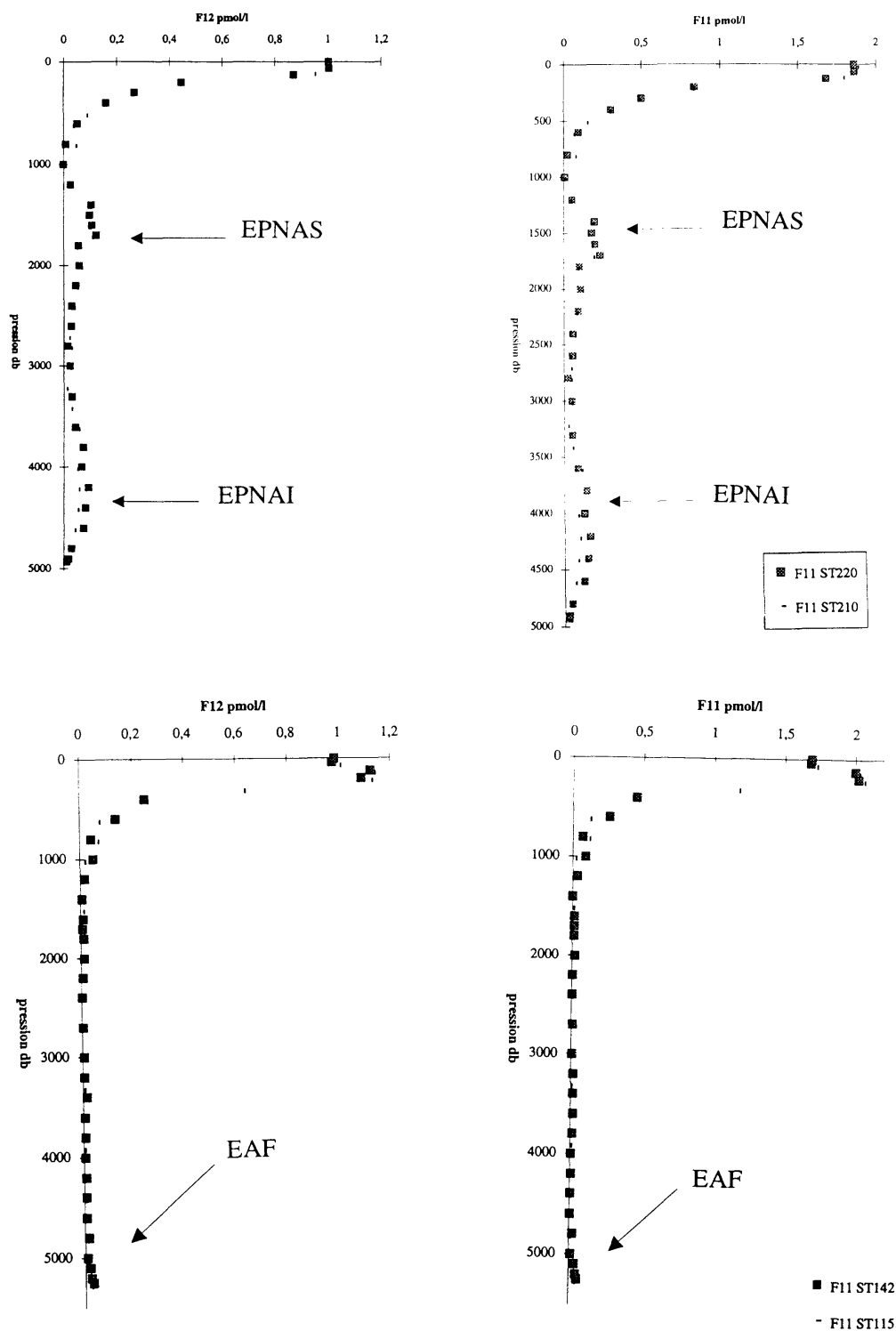
Figure V-4: Profils comparés en données brutes de FI 1 et F12 des stations 142/115 et 210/220 répétées à la même position géographique. On observe: Σ stations 142/115, les signaux de l'Eau Profonde Nord Atlantique Supérieure (EPNAS) vers 1600 dbars et Inférieure (EPNAI) vers 4000 dbars progressant vers le sud Σ stations 210/220, les signaux de L'Eau Antarctique de Fond (EAF) progressant vers le nord vers 5000 dbars de profondeur.
