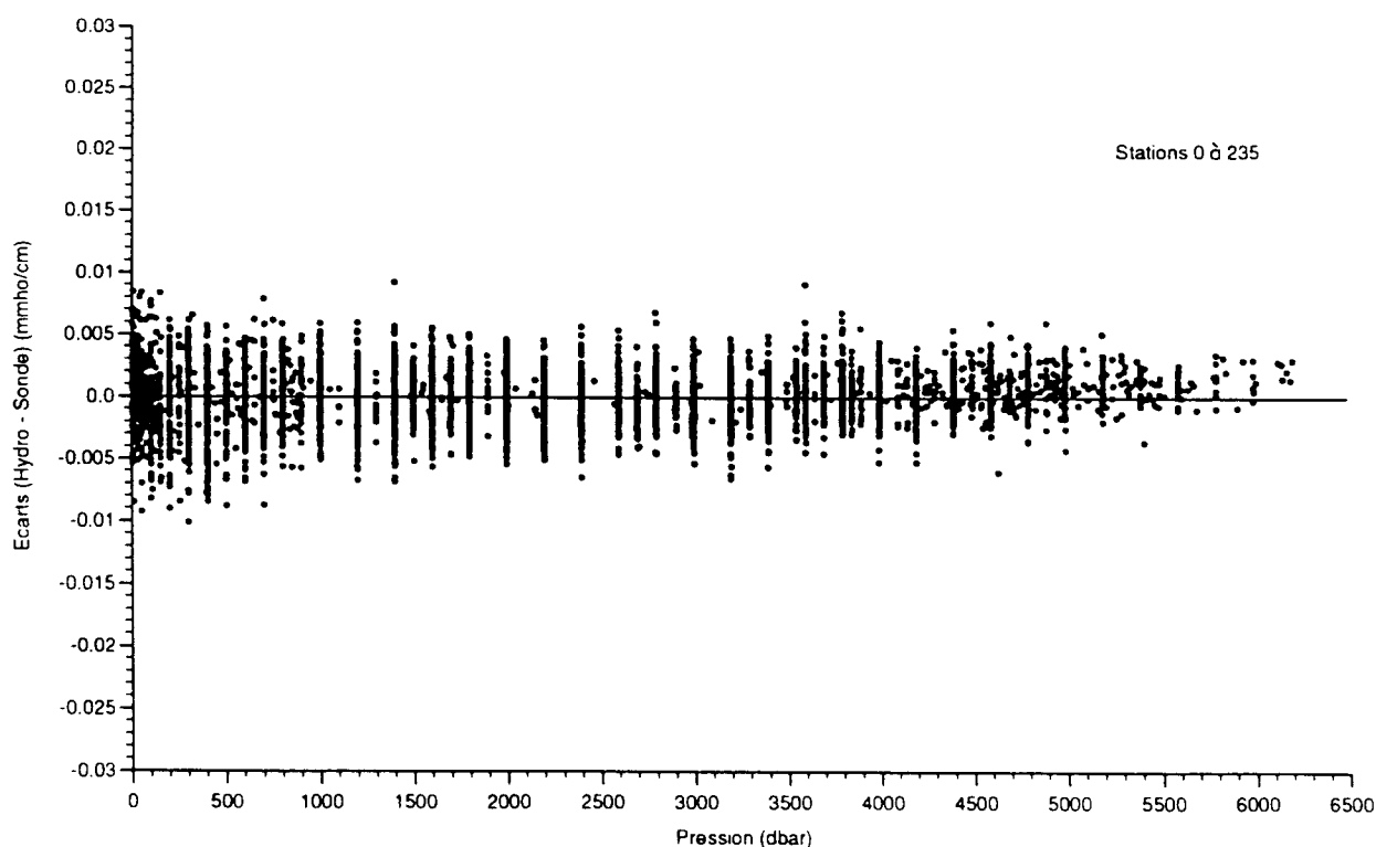
Figure 14: Ecarts entre la conductivité des 5984 échantillons validés et la conductivité "bathysonde", au niveau du prélèvement, après recalage par station ou groupe de stations
