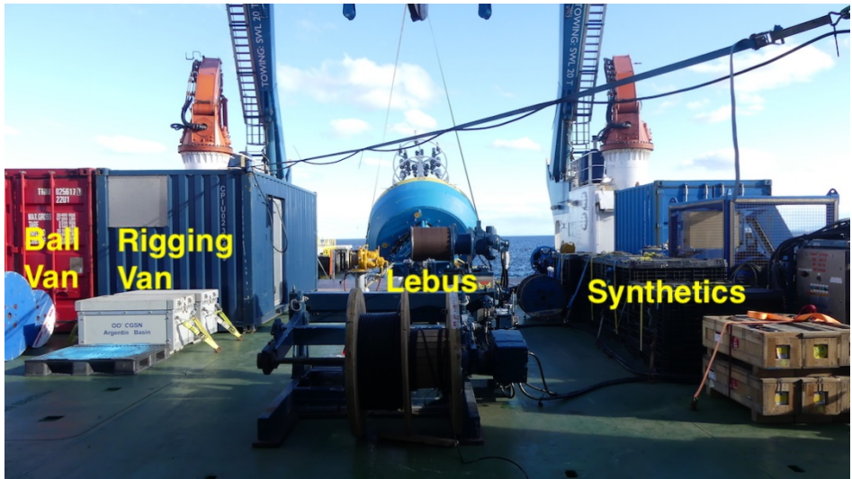
Figure 3 – Actual Deck Layout
